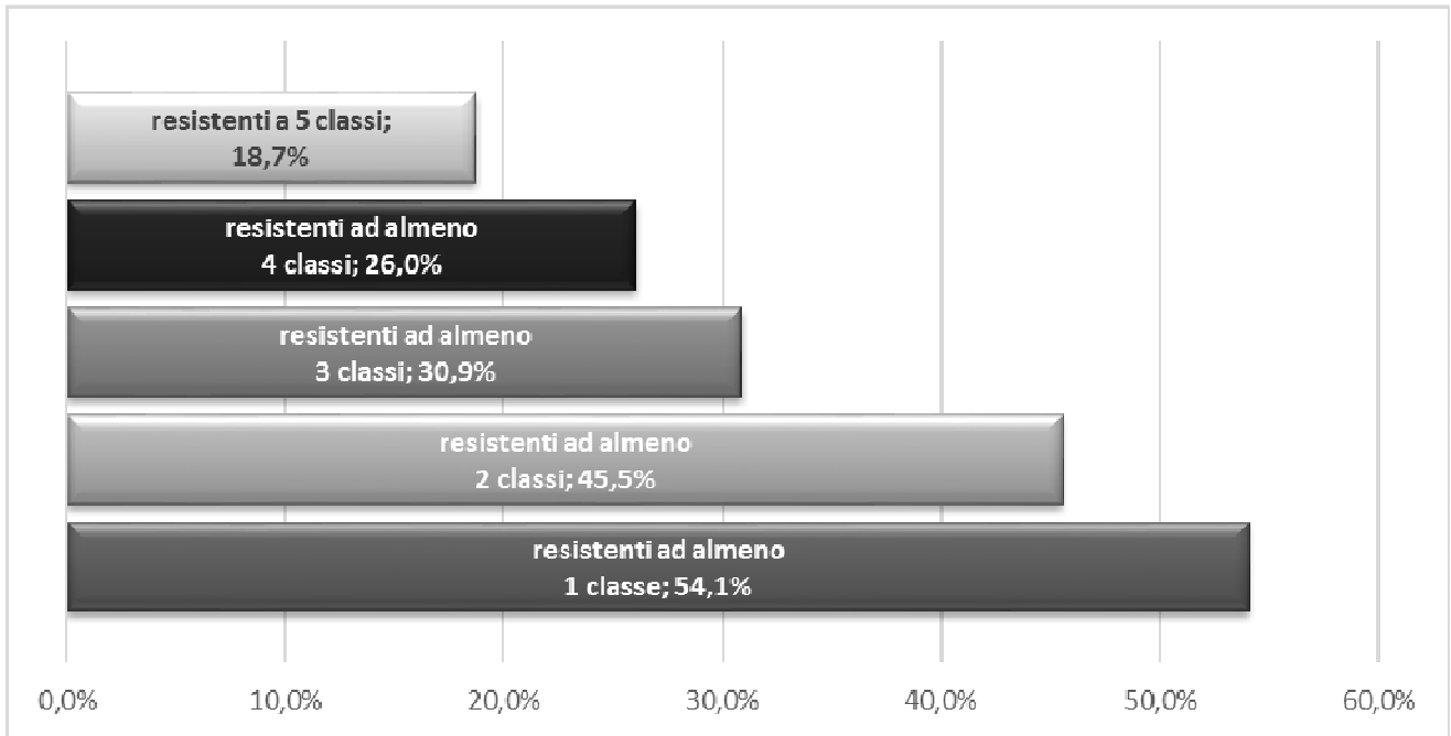
Figura 9. Percentuali di resistenze combinate a Fluorochinoloni, Aminoglicosidi, Carbapenemi, Ceftazidima e Piperacillina+Tazobactam negli isolati invasivi di P. aeruginosa rilevati in Campania nel 2016.
