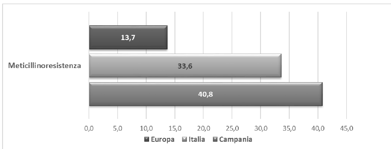
Figura 13. Meticillino-resistenza espressa dagli isolati invasivi di S. aureus : confronto tra le percentuali rilevate nel 2016 in Europa, Italia e Campania.
